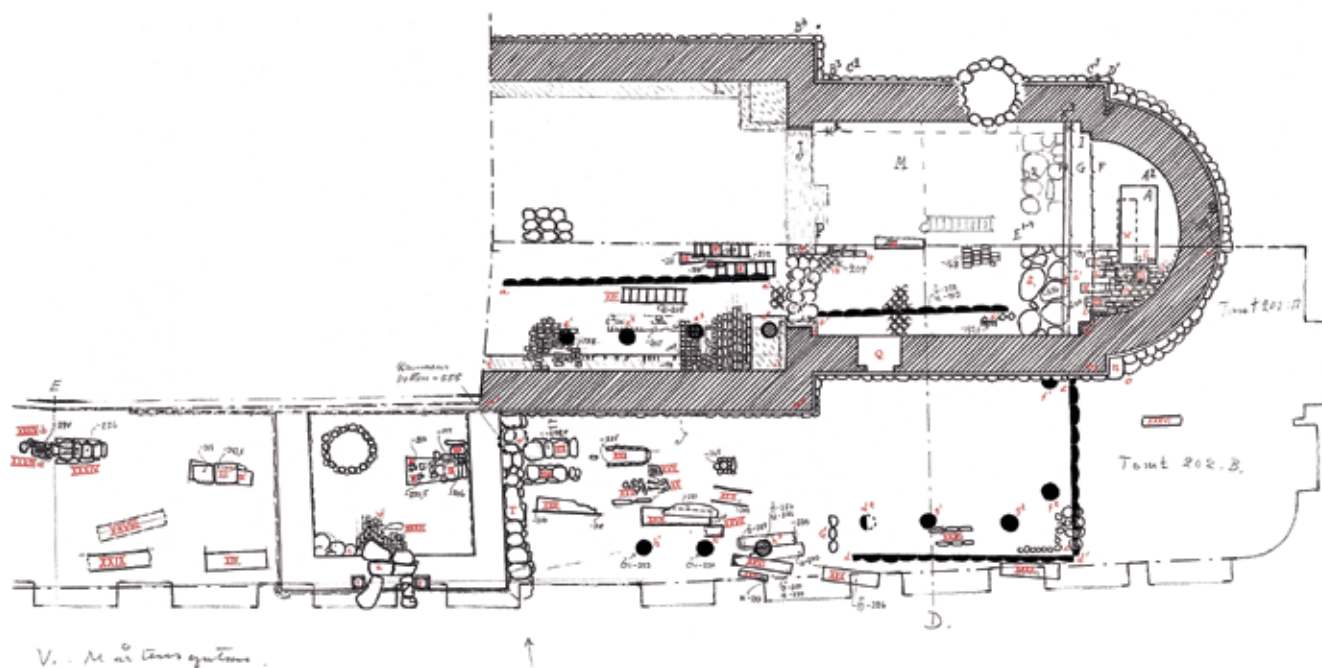
Fig. 23. Planritning över S:ta Maria minors träkyrka och stenkyrka i Lund, gjord i samband med undersökning av kyrkorna 1911–14. Planritning i Kulturens A-arkiv, Lund.
