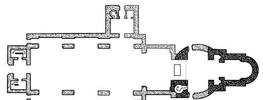
Valleberga, nybyggd 1908-10.
