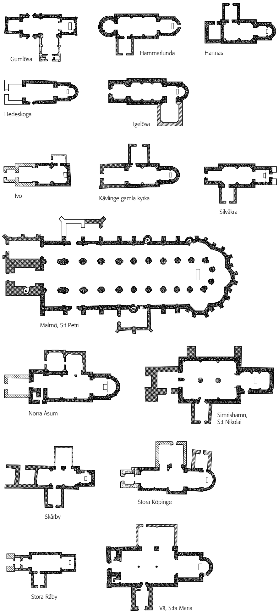
Fig. 34. Ett urval helt eller delvis bevarade kyrkor från äldre medeltid (~1350) i skala 1:800. Planritningarna avser att på ett överskådligt sätt ge en uppfattning om kyrkornas planform, storlek och byggnadshistoria. Förlagorna är vanligtvis hämtade från ritnings-samlingen i ATA. Förlagornas mer detaljerade information har utelutits, däribland fönsteröppningar och innertakets form.
