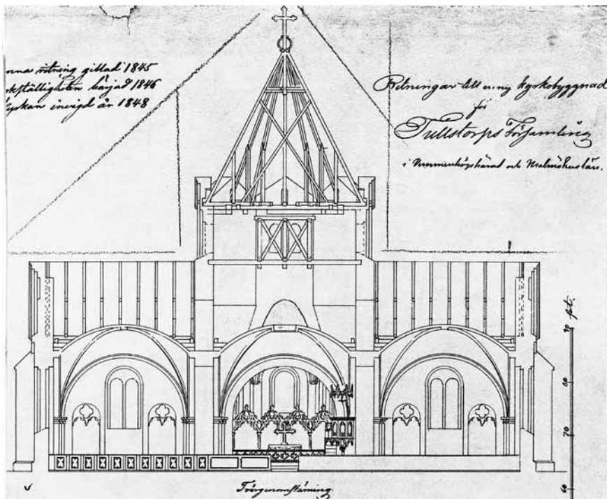
Fig. 115. Carl Georg Brunius, ritning till Tullstorps kyrka 1844, sektion och plan. I den kryssvälvda interiören anas en skärmvägg bakom altaret och en predikstol, bägge med gotiserande bågformer. Inredningen förnyades 1892, men ansluter i stora drag till de ursprungliga idéerna. Foto ATA.
