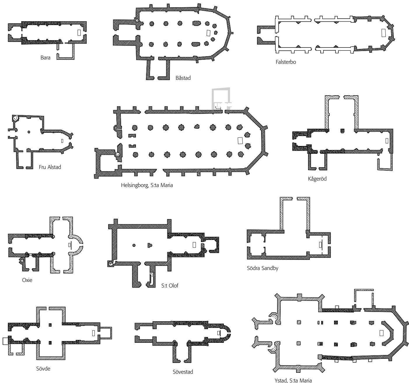
Fig. 64. Ett urval helt eller delvis bevarade kyrkor uppförda eller ombyggda under yngre medeltid (1330–1550) i skala 1:800.
