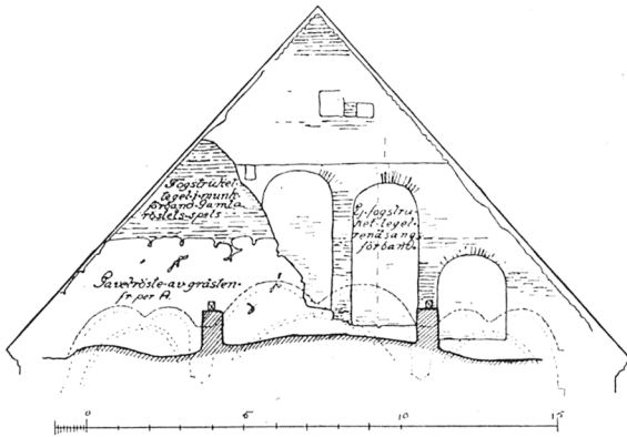
Fig. 15. Danderyd. Östra gavelröstets insida. Uppmätning av prof. L. I. Wahlman.
