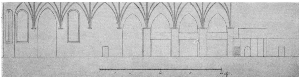
Fig. 218. Längdsektion från 1700-talets förra hälft, visande läktaranordningen i kyrkans södra sidoskepp. B. St. (s. 282).
