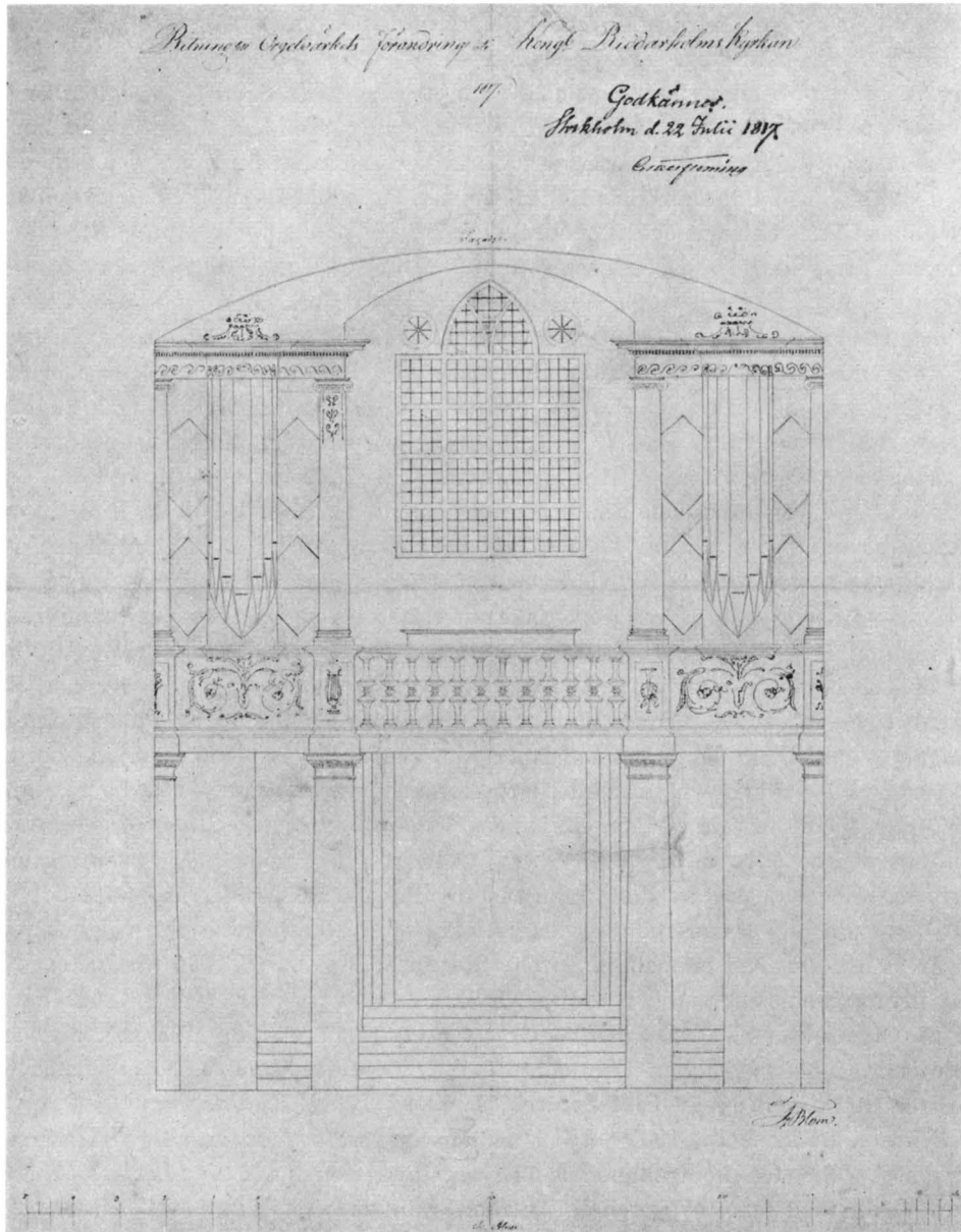
Fig. 215. Ritning till orgellådan av Fredrik Blom 1817. B. St. (s. 270). Entwurf zur Orgellempore von Fredrik Blom (1817). Drawing of organ-loft, by Fredrik Blom, 1817.
