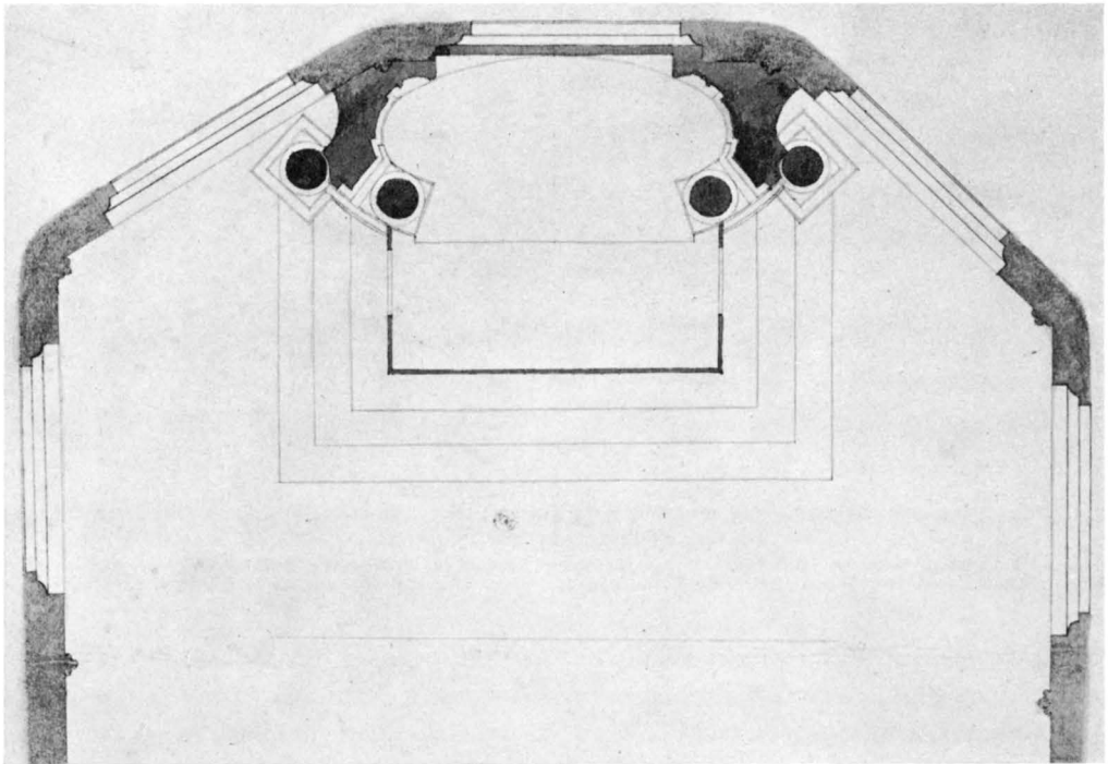
Fig. 209. Plan av högkorets östligaste del med altare, altaruppsats och altarring. Ritning av Nikodemus Tessin d. ä. N. M. (s. 256).
