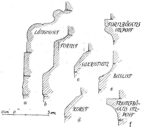
Fig. 453. Endre kyrka. a—d sockelprofiler; e profil av tornbågens impost och bas; f profil av triumfbågens impost.
