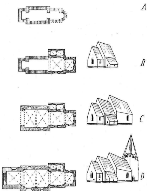
Fig. 591. Barlingbo kyrka. Schematisk utveckling av kyrkobyggnaden.
