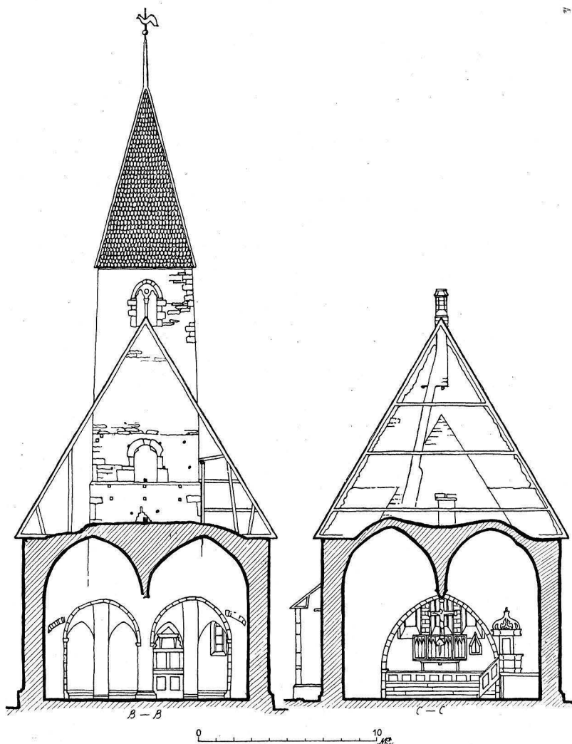
Fig. 450. Endre kyrka. Sektion mot väster och öster. Querschnitt des Langhauses gegen Westen und Osten.
