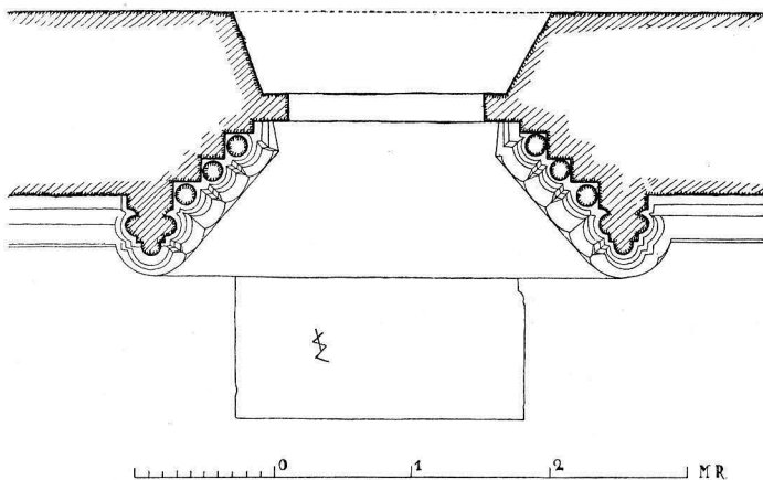
Fig. 459. Endre kyrka. Plan av långhusets sydportal. Grundriss des Langhausportals.
