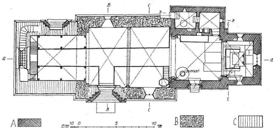
Fig. 551. Barlingbo kyrka. Plan. Grundriss.
