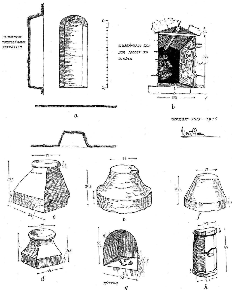
Fig. 431. Hejdeby kyrka. a igenmurat fönster i korets nordvägg; b muröppning mellan tornet och vinden; c, d, e, f kolonnbasen; g piscina; h podium. a Zugemauertes Fenster in der Nordwand des Chores; b Maueröffnung zwischen Turm und Langhausoberboden; c, d, e, f Säulenbasen; g Piscina; h Podium.
