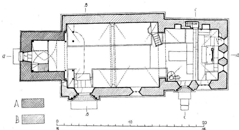
Fig. 506. Ekeby kyrka. Plan. Grundriss.
