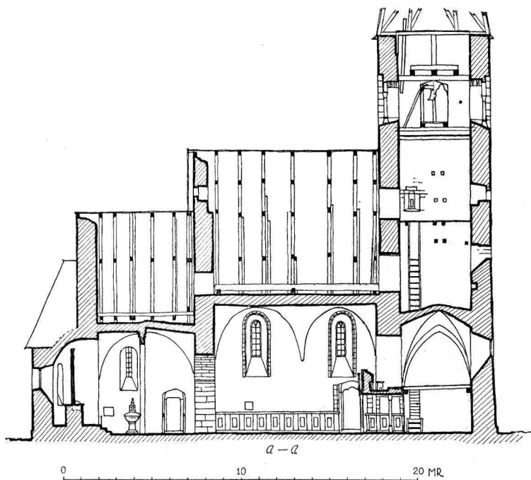
Fig. 422. Hejdeby kyrka. Längdsektion mot söder. Längsschnitt gegen Süden.
