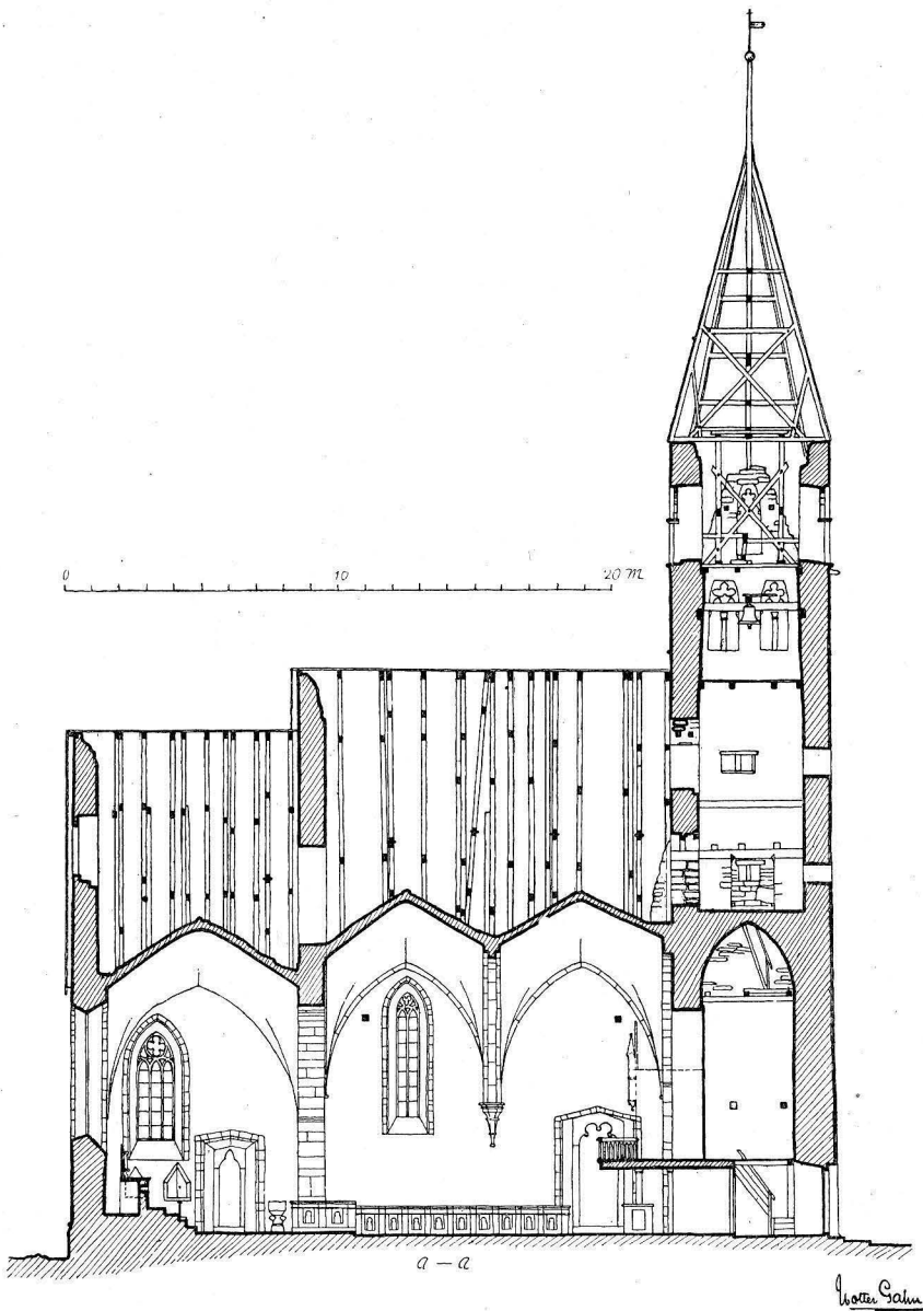
Fig. 509. Ekeby kyrka. Längdsektion mot söder. Längsschnitt gegen Süden.
