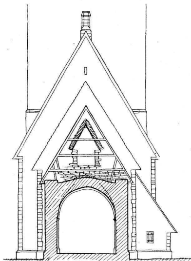
Fig. 547. Barlingbo kyrka. Tvärsektion av koret. Querschnitt des Chores.
