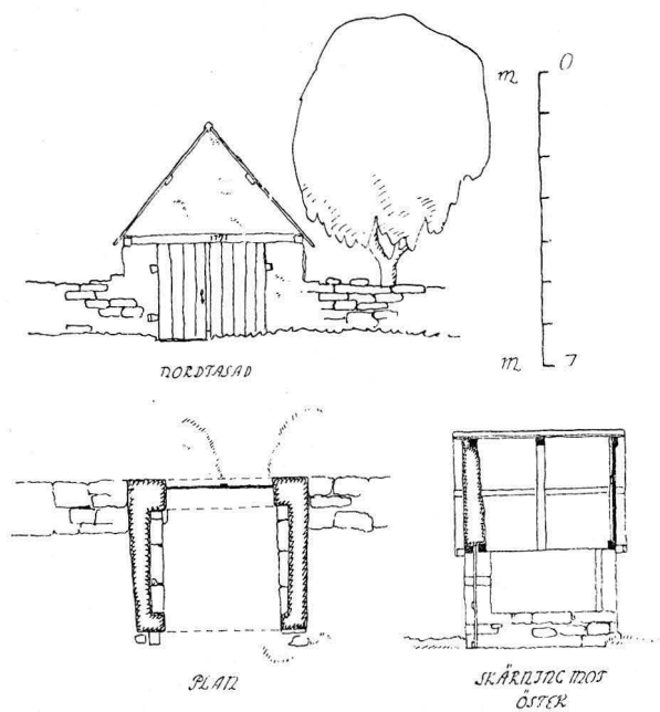
Fig. 505. Ekeby kyrka. Uppmätning av kyrkogårdsportalen fig. 504. Abmessung des Friedhofsportals Fig. 504.
