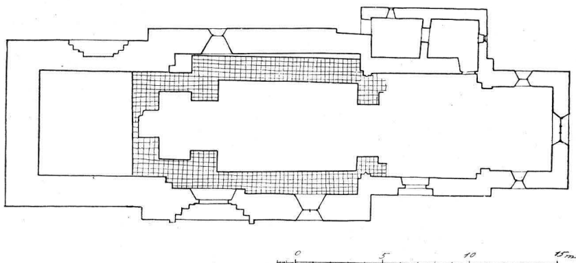
Fig. 552. Barlingbo kyrka. Plan med intecknade äldre grundmurar, funna vid grävning.
