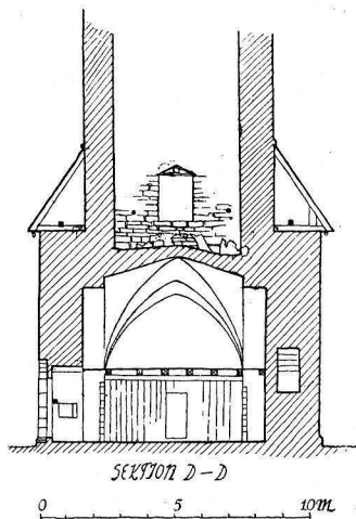
Fig. 426. Hejdeby kyrka. Tornsektion.
