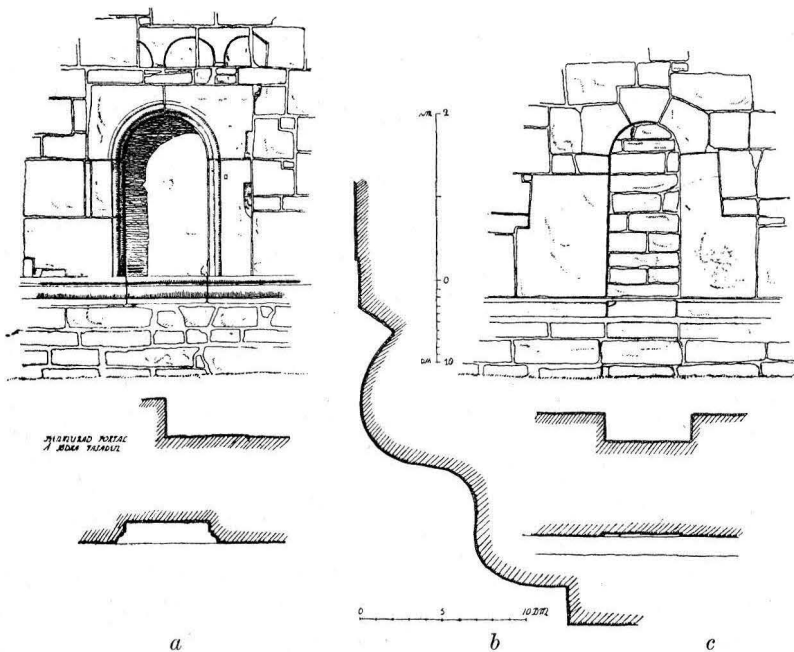
Fig. 456. Endre kyrka. a Penitenscellens portal; b profil av portalen fig. a c tornportal.
