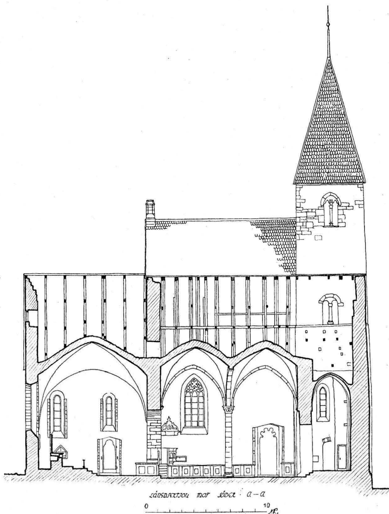
Fig. 451. Endre kyrka. Längdsektion mot söder. Längsschnitt gegen Süden.
