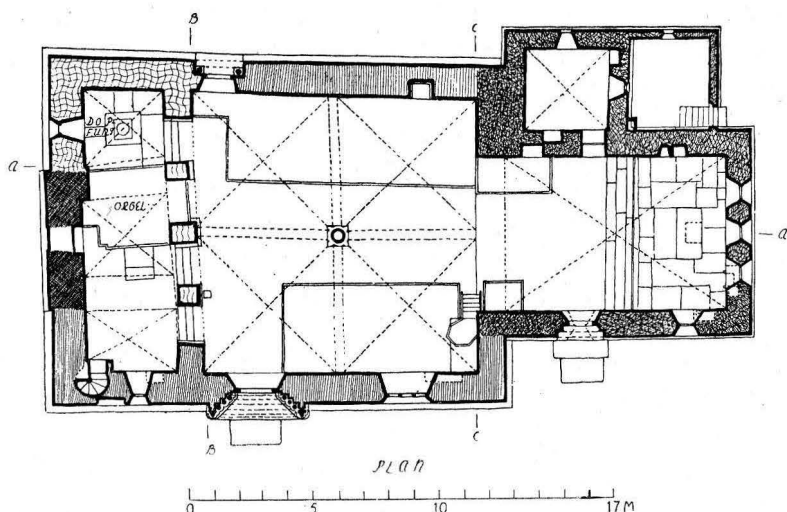
Fig. 448. Endre kyrka. Plan. Grundriss.
