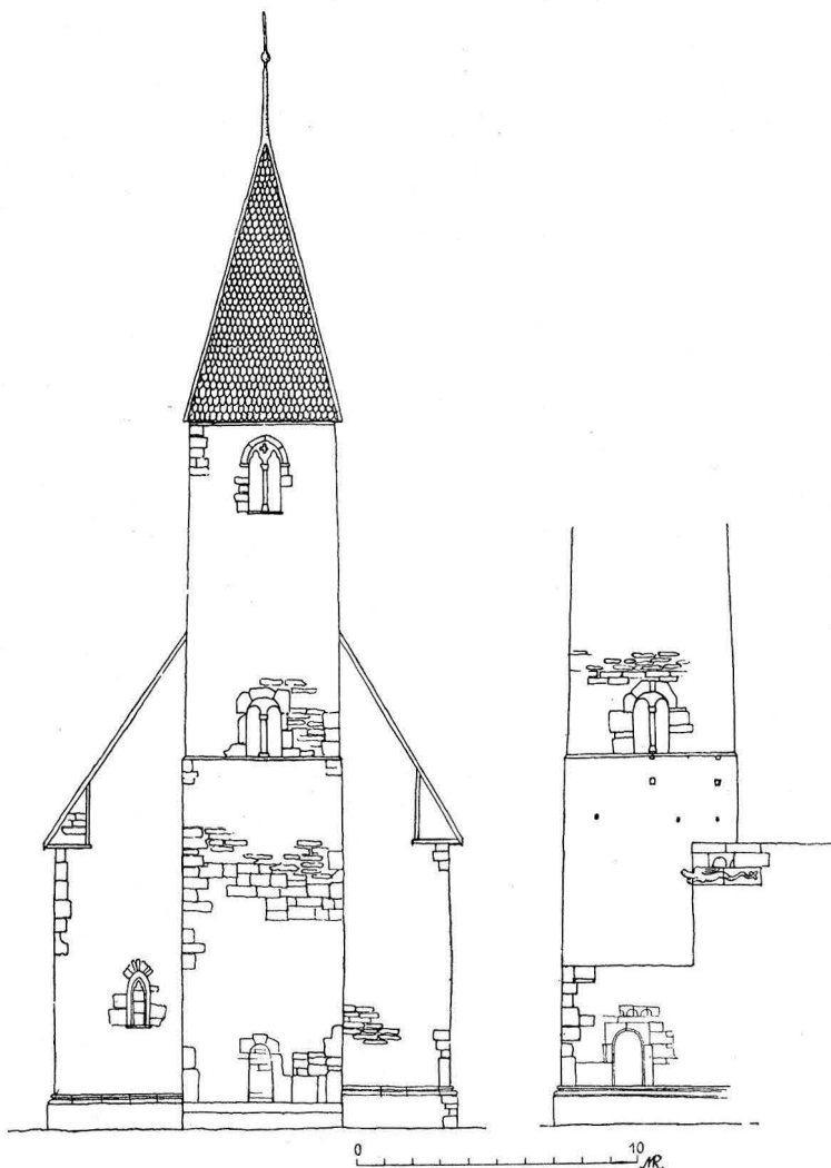
Fig. 452. Endre kyrka. Uppmätning av västfasaden samt västligaste delen av sydfasaden; botgöringscellens ursprungliga höjd är markerad på högra bilden (jfr s. 409).
