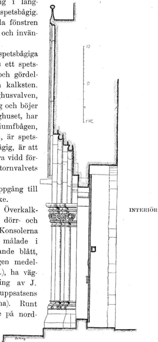
Fig. 511. Ekeby kyrka. Sektion av långhusportalen.
