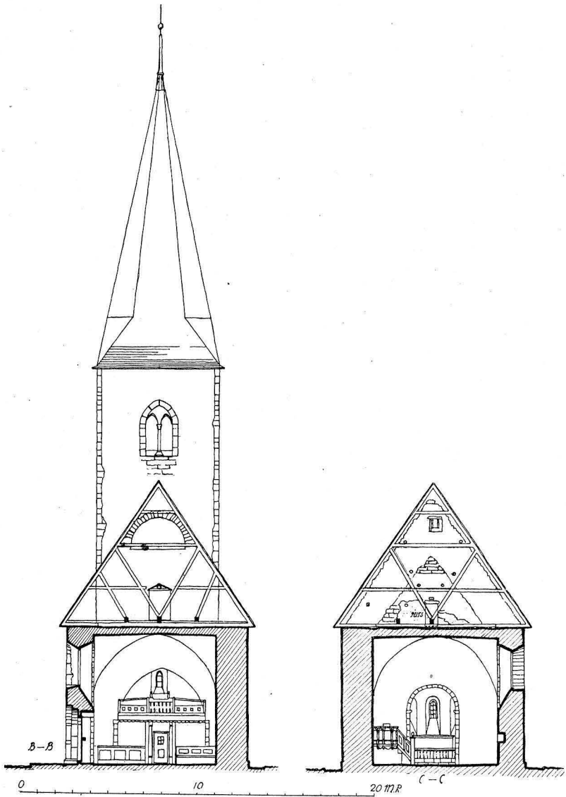
Fig. 424. Hejdeby kyrka. Tvärsnitt genom långhuset mot väster och mot öster. Querschnitt durch das Schiff gegen Westen und Osten.
