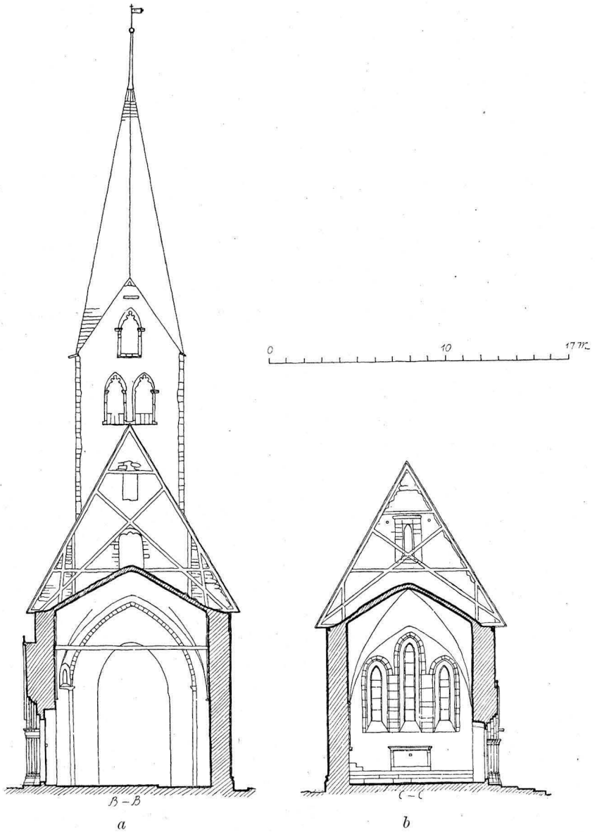
Fig. 508. Ekeby kyrka. Tvärsektion a mot väster och b mot öster. Querschnitte; a gegen Westen, b gegen Osten.
