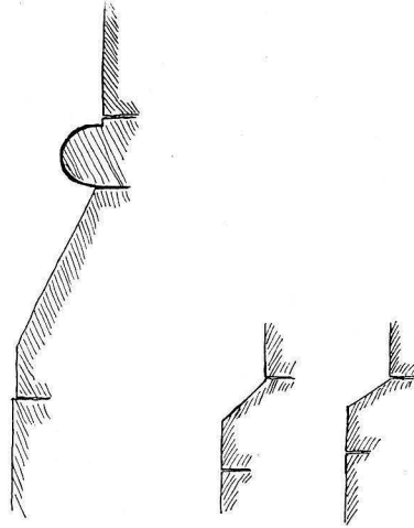
Fig. 507. Ekeby kyrka. Sockelprofiler. Sockelprofile.
