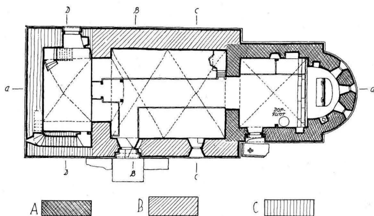
Fig. 423. Hejdeby kyrka. Plan. Grundriss.
