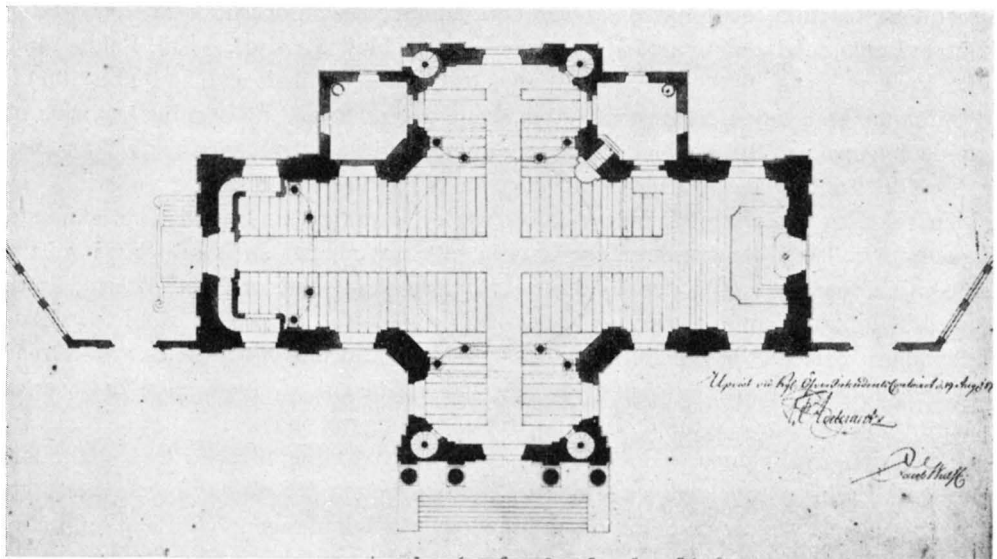
Fig. 219 a, b . Sydfasad och plan av J. E. Rehns första förslag till ny kyrka i St. Johannes 1780. Erster Vorschlag zu einer neuen Kirche in St. Johannes von J. E. Rehn 1780. Südfassade und Grundriss. J. E. Rehn's first project for a new church in St. Johannes 1780. Plain, front and plan.
