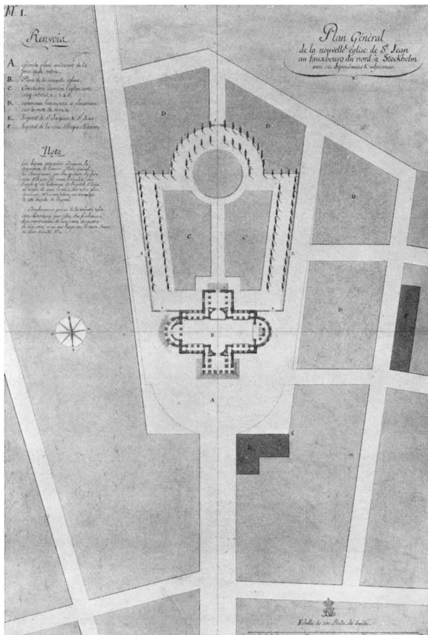
Fig. 224. Léon Dufourny's projekt till kyrka och kyrkogård 1784.
