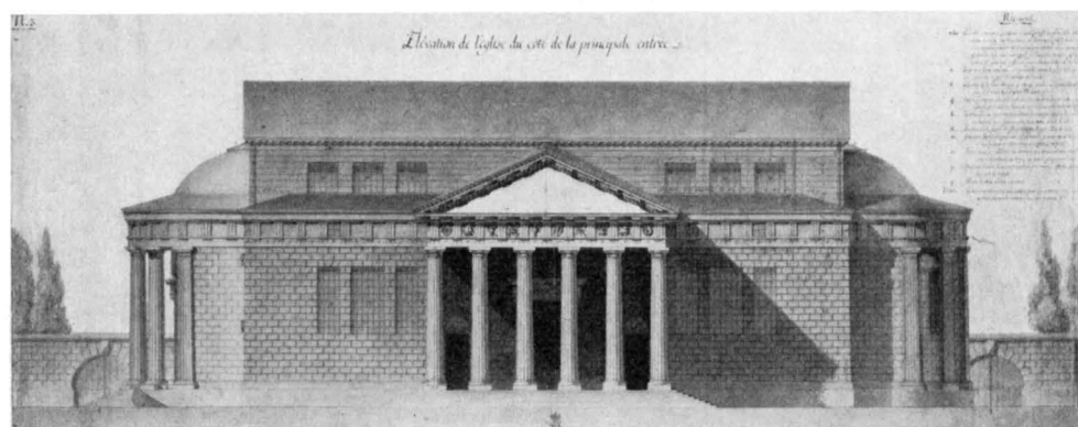
Fig. 225 a, b. Plan och sydfasad av Dufourny's kyrkoförslag 1784. Grundriss und Haupt(süd-)fassade. Von Dufourny 1784. Plan and main front of the church as projected by Dufourny 1784.
