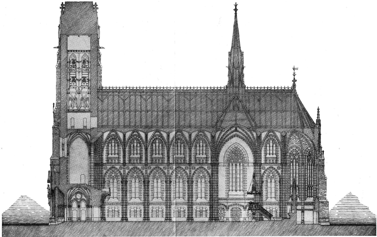
St Johannes kyrka. Längdsektion mot öster. Efter Carl Möllers originalritning. Skala 1:400.
