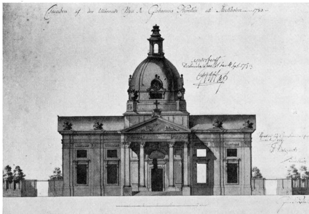
Fig. 216. Förslag till ny kyrka i Johannes av J. E. Rehn, antaget 1783. Huvudfasad. Der 1783 approbierte Vorschlag zu einem neuen Kirchenbau von J. E. Rehn. Hauptfassade. Project for a new church by the architect J. E. Rehn. 1783. Main front.
