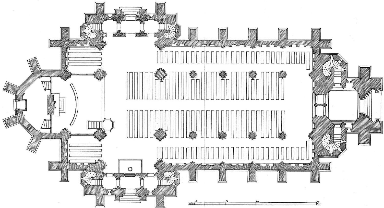
St Johannes kyrka. Plan. Skala 1:300. (E. Ullrich 1933). Grundriss der Johanneskirche. Plan of St. Johannes' church.
