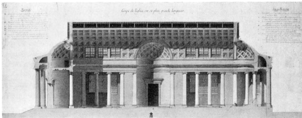
Fig. 226 a—c. Västfasad, tvär- och längdsektion enl. Dufourny's förslag 1784. West facade, cross- and longitudinal section of the church as projected by Dufourny 1784.
