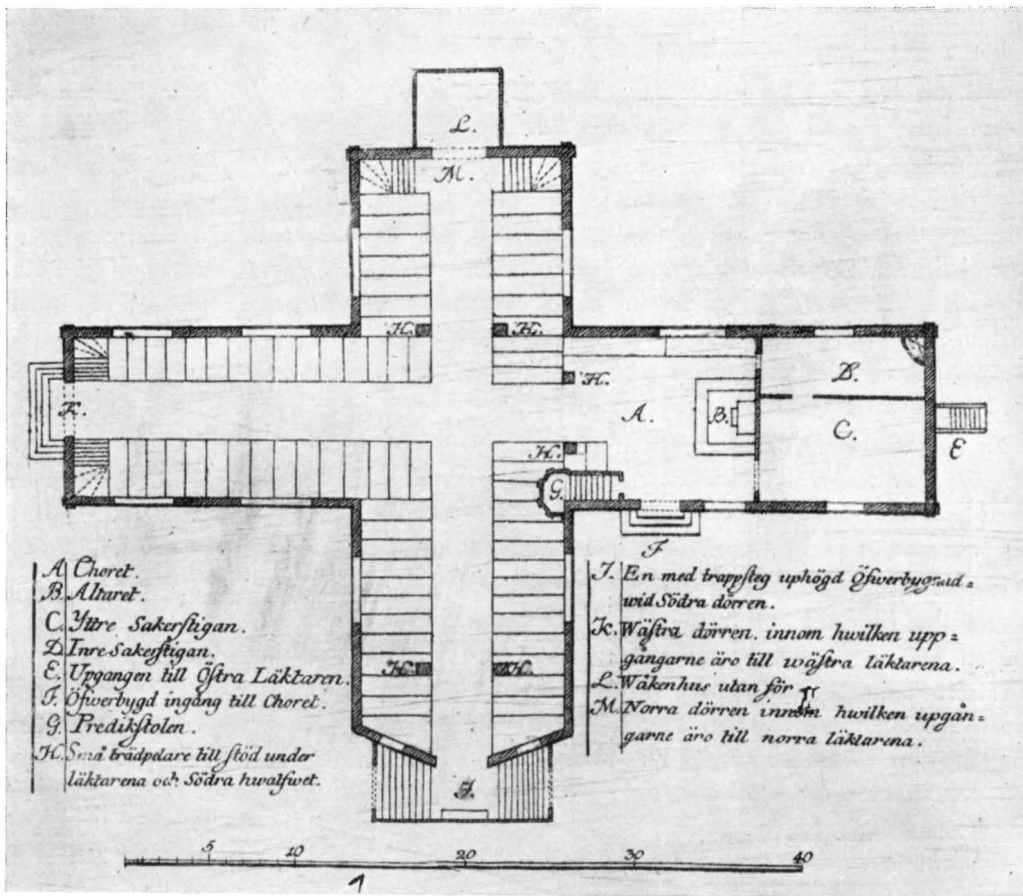
Fig. 214. Johannes kapell. Plan enl. WITTING.
