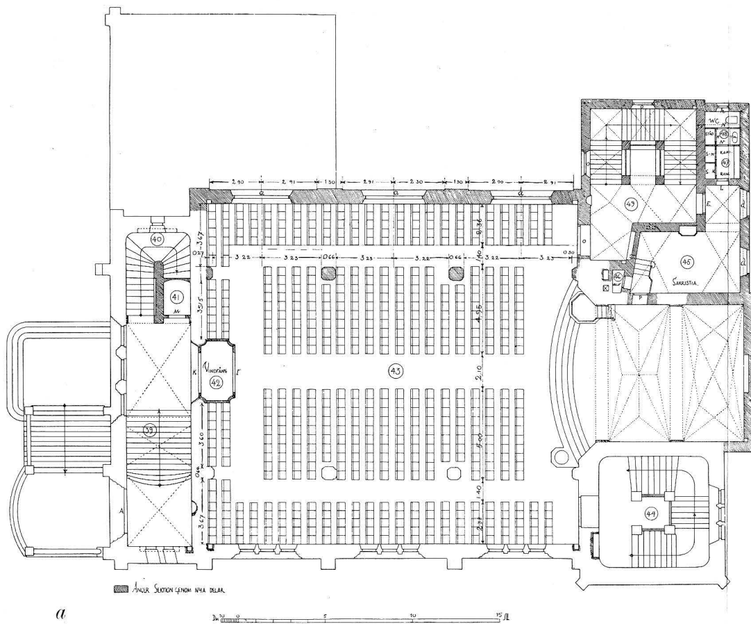
Plan (a) och längdsektion (b) mot öster av S:t Stefans kapell. Skala 1:300.
