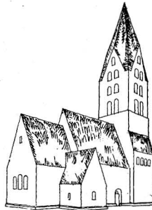
Fig. 196. Tingstäde kyrka. Schematisk utveckling. Haupt-etappen in der baugeschichtlichen Entwicklung der Kirche.
