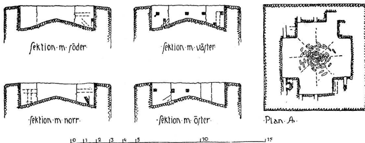
Fig. 160. Tingstäde. Plan och sektioner av tornet i höjd med det övre valvets hjässa.
