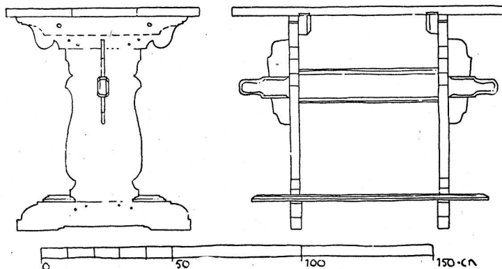
Fig. 192. Tingståde. Bord. 1600-talet. Tisch. 17. Jht.
