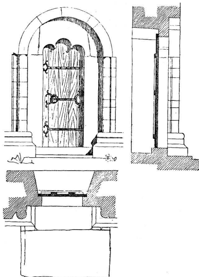
Uppmätning av Leche och Westerberg. Fig. 142. Tingstäde. Långhusets nordportal. Skala 1:80. Nordportal des Langhauses.
