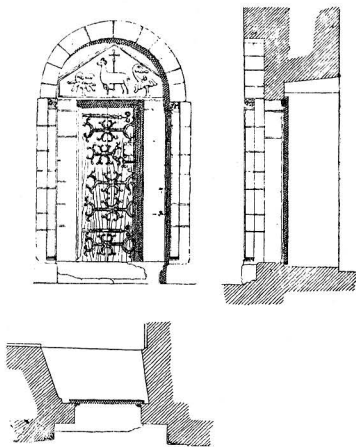
Fig. 151. Tingstäde. Sakristiportal, förut portal till äldre kor.
