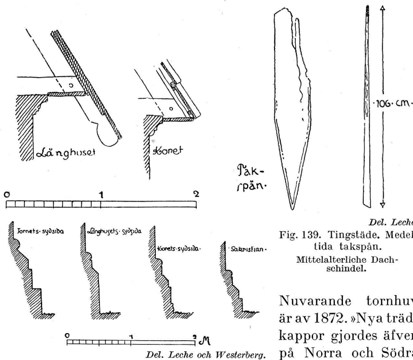
Fig. 138. Tingstade. Taklist- och sockelprofiler. Dachgesims- und Sockel-Schnitte.
