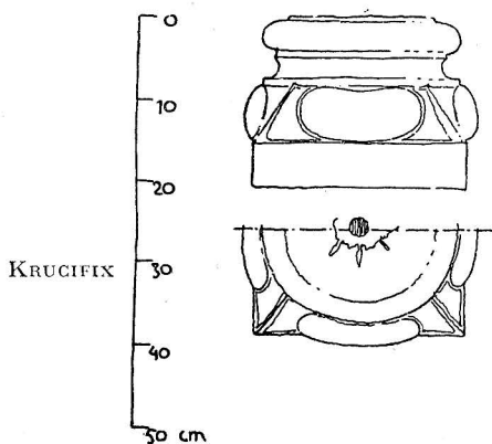
Fig. 171. Tingstäde. Bas till piscina. 1100-talets senare hälft. Unterer Teil einer Piscina. 2. Hälfte d. 12. Jhts.
