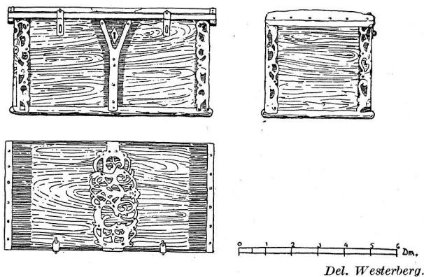
Fig. 194. Tingstäde. Kista. 1600-talet.
