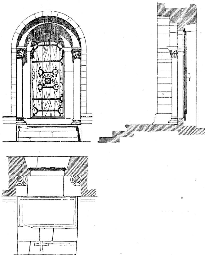
Fig. 140. Tingstäde. Långhusets sydportal, fasad, plan och sektion.
