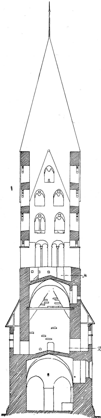
Fig. 159. Tingstäde. Sektion genom tornet mot öster.
