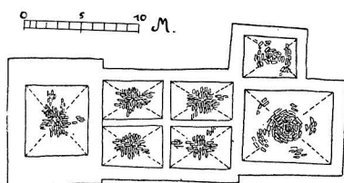
Del. Leche och Westerberg. Fig. 143. Tingstäde. Valvschema. Schema der Gewölbekonstruktion.
