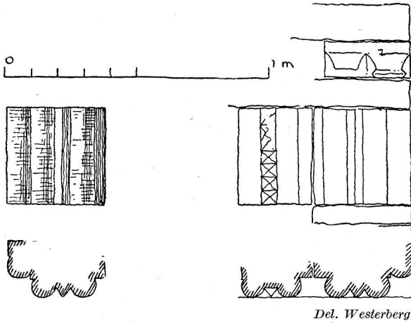
Fig. 133. Tingståde. Huggna stenar i norra kyrkogårdsportalen. Omkr. 1260.
