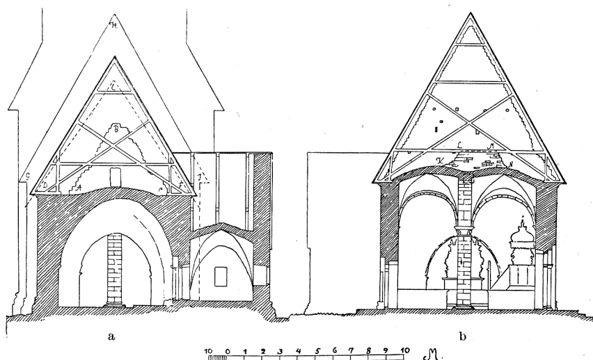
Fig. 165. Tingstade. a koret och sakristian, tvärsnitt mot väster; b långhuset, tvärsnitt mot öster.
