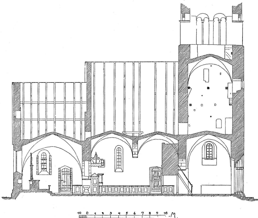
Fig. 158. Tingstade. Längdsektion mot söder. Längsschnitt gegen Süden.
