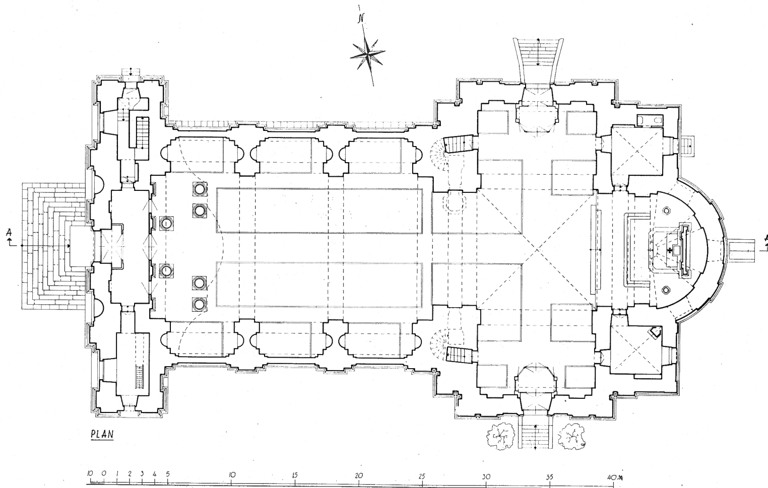
Fig. 7. Plan. Grundriss. Plan.
