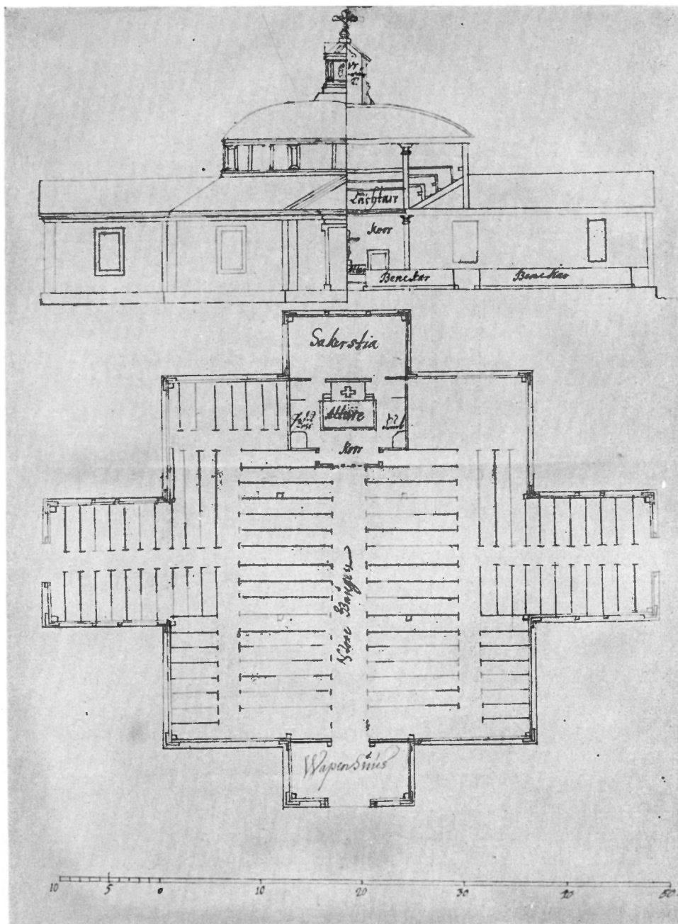
Fig. 3. Hedvig Eleonora kyrka enl. uppmätning.
