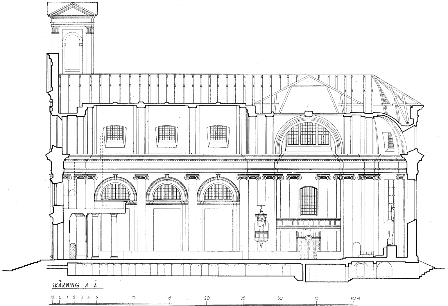
Fig. 6. Längdsektion mot norr. Längsschnitt gegen N, Longitudinal section facing N.
