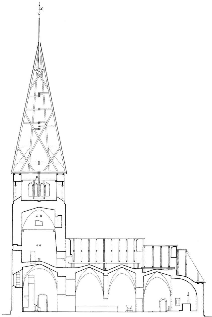
SKÄRNING A-A
