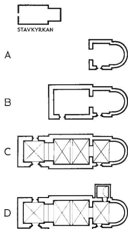
Fig 305. Kyrkans planutveckling, 1 : 1000.
