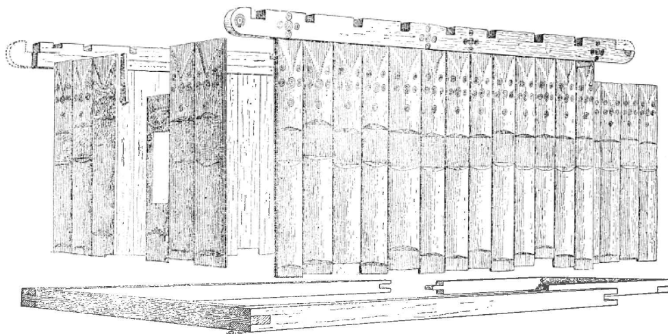
Fig 208. Försök till rekonstruktion av stavkyrkans exteriör. Efter Ekhoff. Suggested reconstruction of exterior of stave church.
