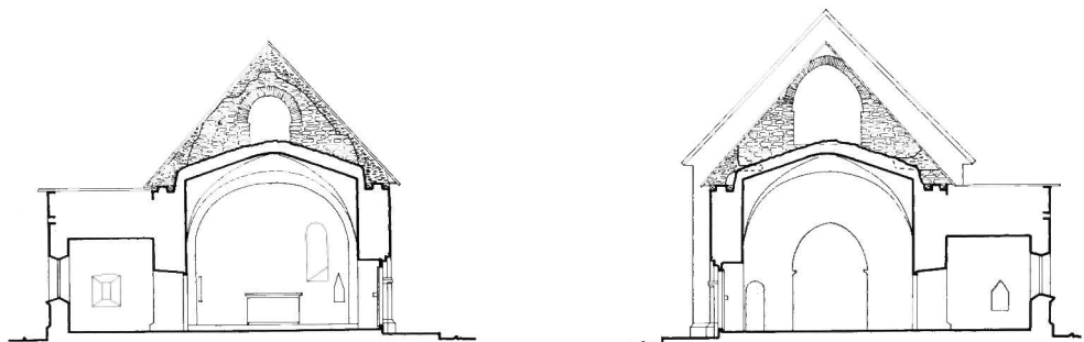
Fig 212. Sektioner av koret mot öster och väster, 1:300. Uppm J Söderberg 1943-44 och 1967. Sections of chancel looking E and W.
