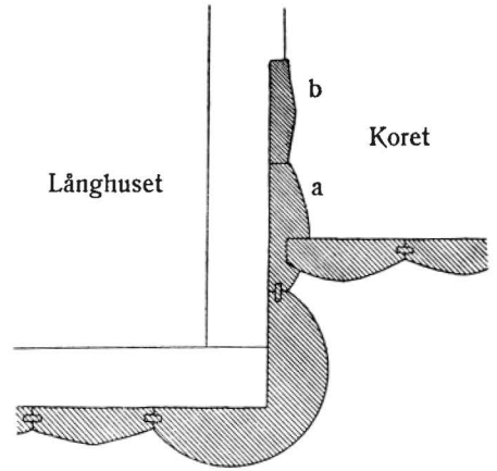
Fig 204. Förmodad konstruktion av stavkyrkans hörn. Efter Ekhoff.
