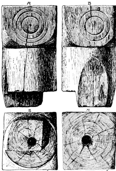
Fig 202. Tärningskapital av furu, från stavkyrkan. Efter Ekhoff.
