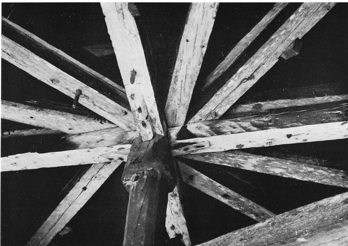
Fig 229. Detalj av tornspirans stödkonstruktion. Foto 1967. Detail of construction of spire.
