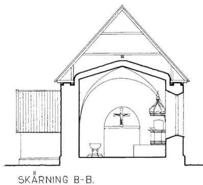
Fig 212 a. Sektion av långhuset mot öster. Uppm J Söderberg 1943-44.
