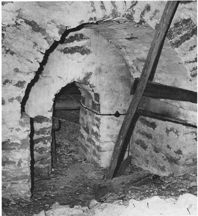
Fig 226. Avlastningsbåge samt ingång till långhusvinden i tornets första våning. Foto 1967.
