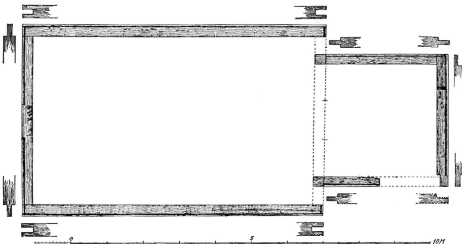
Fig 206. Stavkyrkans rekonstruerade plan. Efter Ekhoff.
