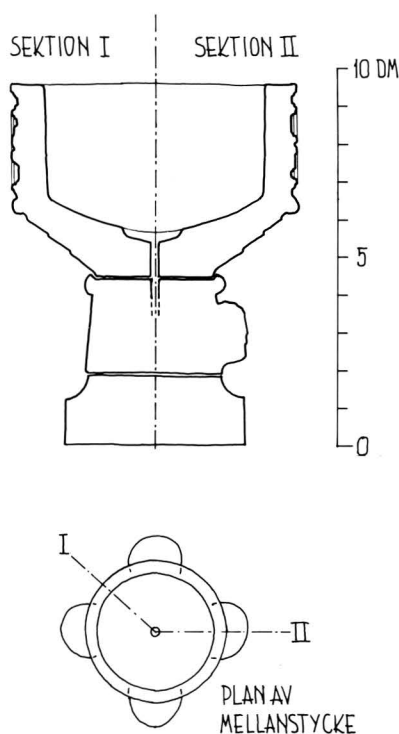
Fig 98. Sektioner av dopfunten samt plan av mellanstycket. Skala 1:20, uppm S Hesselgren & S Fränne 1931, kompl R Boström 1979.
