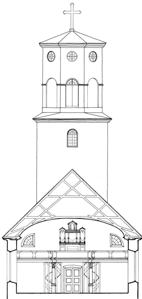
SEKTION MOT VÄSTER
