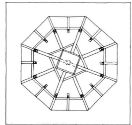
LANTERNINTAKSTOL.
