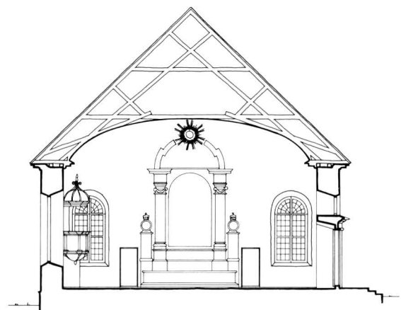
SEKTION MOT ÖSTER
