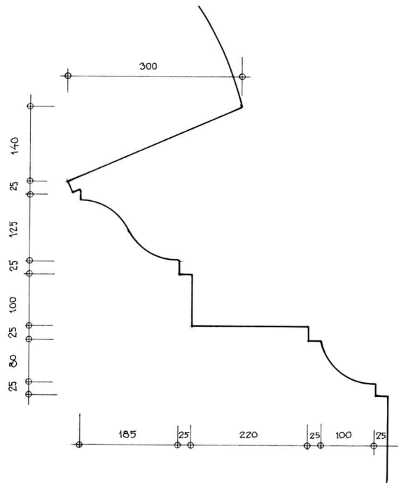
Fig 76. Taklistprofil. Uppm, skala 1 : 10, G Wirén 1978.
