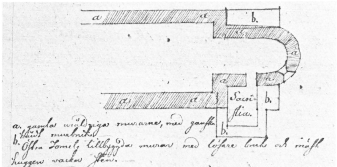
Fig 25. Plan av den medeltida kyrkans östra del. Teckning av A Ahlqvist 1836 (RM, VaLA).
