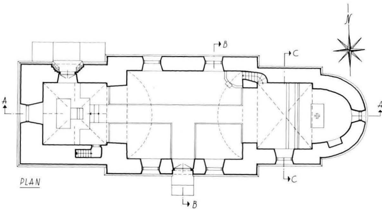
Fig 15. Plan, längdsektion mot norr, 1:300, samt kapitäl från den rivna långhuskolonnen, 1:30. Uppm J Söderberg 1943.
