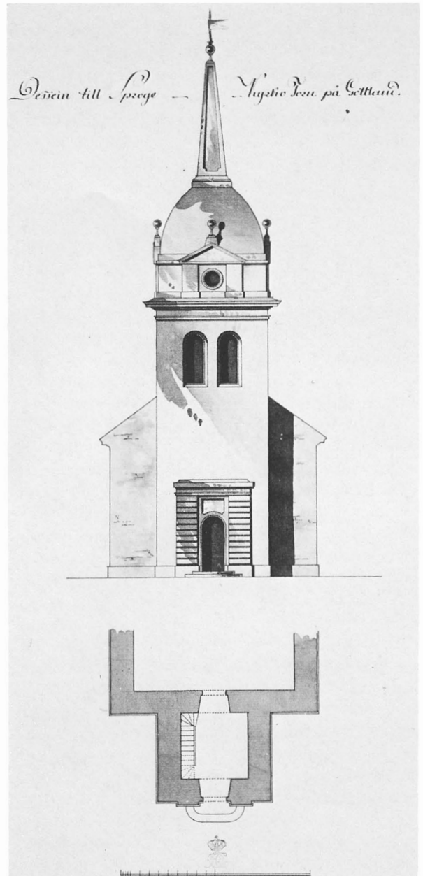
Fig 36. Förslagsritning till tornets ombyggnad av T G Wennberg 1780, i ÖIÄ:s ritningsarkiv, RA. Foto RA.
