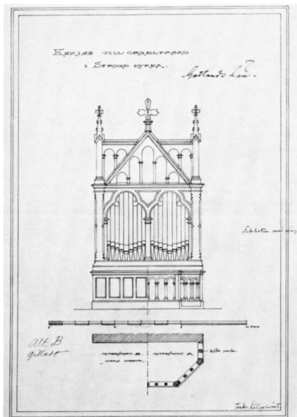
Fig 62. Ritning till orgelfasad av F Lilljekvist 1892, i ÖIÄ:s ritningssamling, RA. Foto RA.
